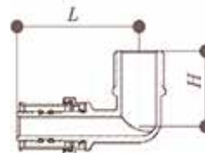
Угольник пресс-резьба, 8006 Aquasfera
