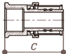
Соединитель пресс-муфта, 8002 Aquasfera
