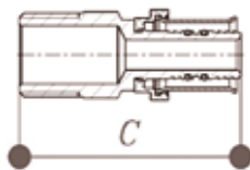
Соединитель пресс-резьба, 8001 Aquasfera
