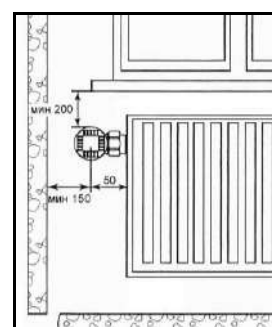
Рис. 5.5. Размещение терморегулятора
